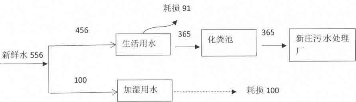
图 3.3-1 项目水平衡图 t/a
